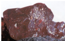
Metacinnabarit
